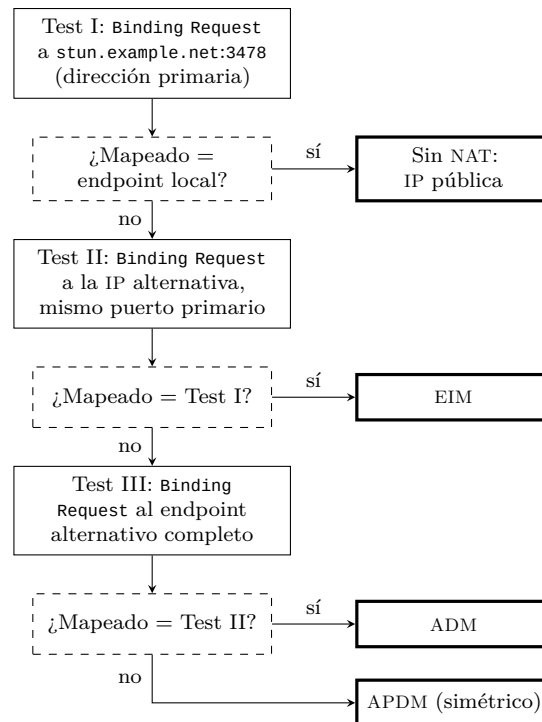
FIGURA 11.9: Determinación del tipo de mapeado NAT con STUN
